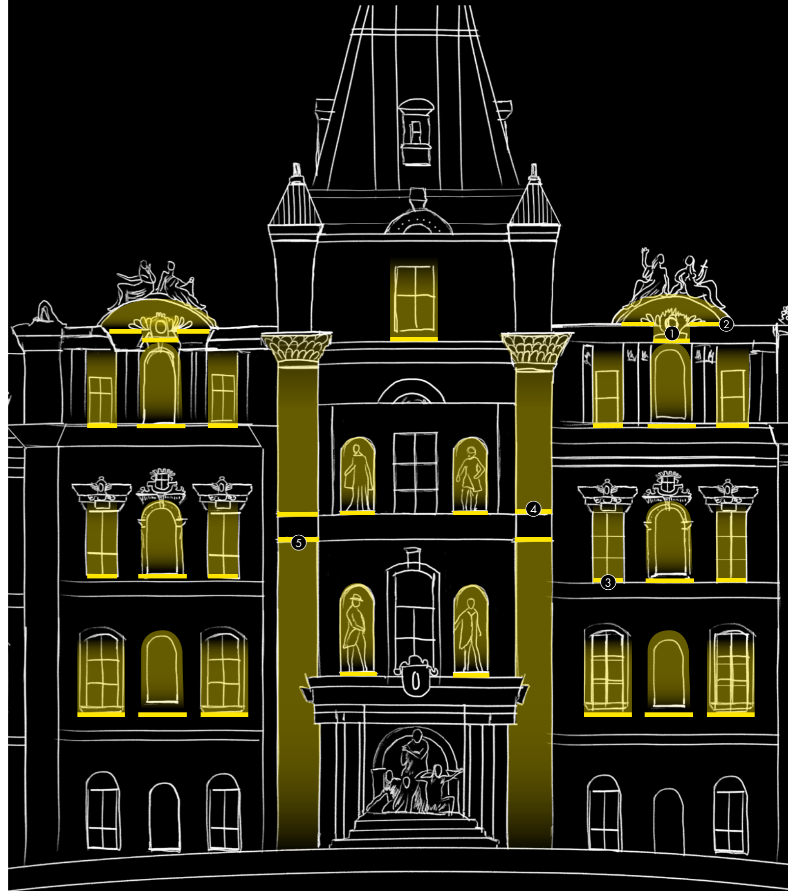
1. Lumenfacade Nano 2W 10°x60° 2. Lumenfacade Nano 4W Wallwash 3. Lumenfacade Nano 4W 10°x30° 4. Lumenfacade Nano 7W 10°x30° 5. Lumenfacade Nano 7W 10°x10°
